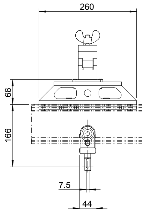
Half Coupler Abhängung und 2-Rad-Laufwagen / Suspension collier et chariot simple / Suspension Bracket for Half Coupler and 2-Wheel Runner
