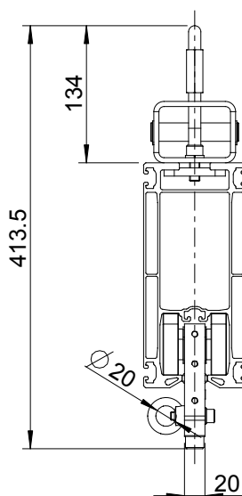
Ringösenabhängung und Scheinwerferlaufwagen / Suspension maillon rapide et conducteur pour projecteur / Eye Style Suspension Bracket and Studio Runner
