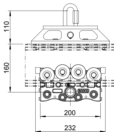
Ringösenabhängung und 2-Rad-Laufwagen / Suspension maillon rapide et chariot simple / Eye Style Suspension Bracket and 2-Wheel Runner
