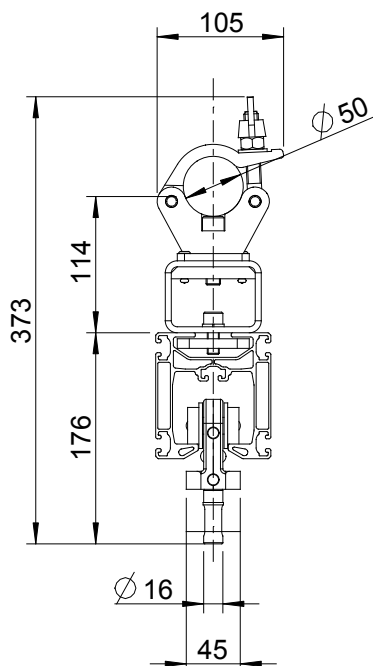
Half Coupler Abhängung und 2-Rad-Laufwagen / Suspension collier et chariot simple / Suspension Bracket for Half Coupler and 2-Wheel Runner
