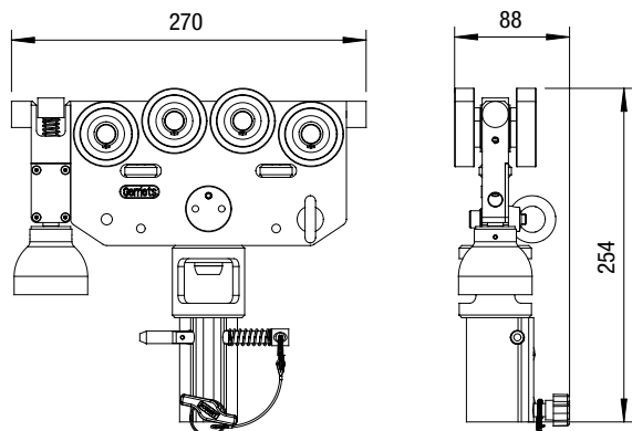
Scheinwerferlaufwagen TV-Zapfenaufnahme – Rastbremse / Conducteur avec support pour projecteur et frein avec ressort de repos / Studio Runner 3-Point Spigot Receiver – Rest Brake
