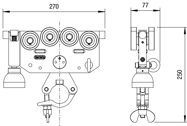
2-Punkt-Traversenlaufwagen mit Federbremse / Chariot pour échelle avec frein à ressort / 2-Point Truss Runner with Spring Brake
