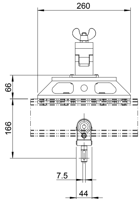
Half Coupler Abhängung und 2-Rad-Laufwagen / Suspension collier et chariot simple / Suspension Bracket for Half Coupler and 2-Wheel Runner
