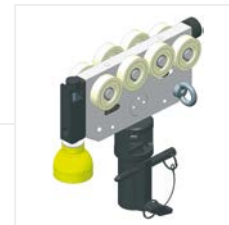
31280 00312 Scheinwerferlaufwagen TV-Zapfenaufnahme – Federbremse / Conducteur avec support pour projec- teur et frein   ressort / Studio Runner 3-Point Spigot Receiver – SWL Screw Brake
