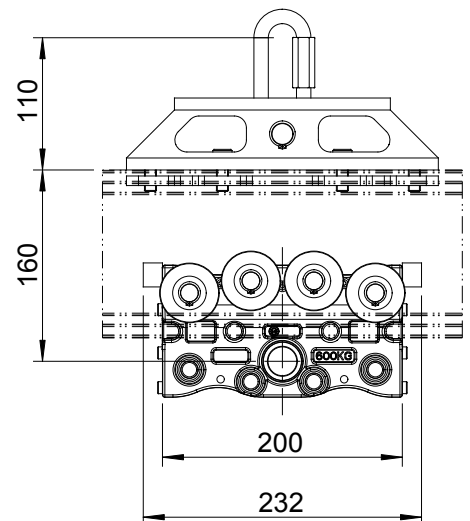
Ringösenabhängung und 2-Rad-Laufwagen / Suspension maillon rapide et chariot simple / Eye Style Suspension Bracket and 2-Wheel Runner
