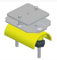
31280 09051 Endklemme Flachkabel / Bride d'arrêt pour câble plat / Fixed End for Flat Cable
