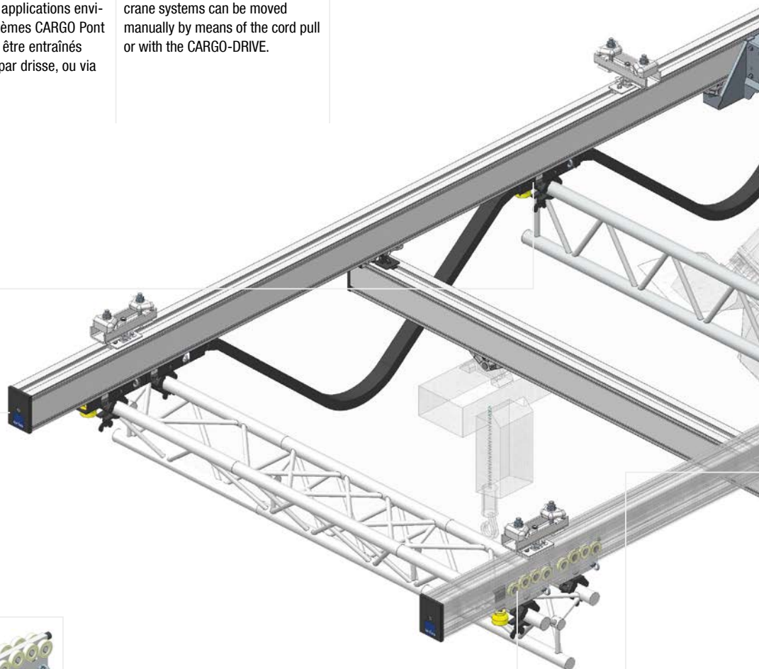
31280 00571 / 00572 3-/4-Punkt-Traversenlaufwagen-Set mit Schraubbremse und Energiekettenaufnahme / Chariot pour Traverse 3-/4 points avec frein à visser et support pour chaîne porte-câbles / 3-/4-Point Traverse Runner with Screw Brake and Energy Chain Adaptor
