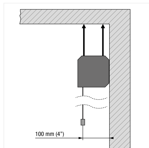
Aufbau E: Seitenansicht / Configuration d'essai E: Vue latérale / Application E: Side View
