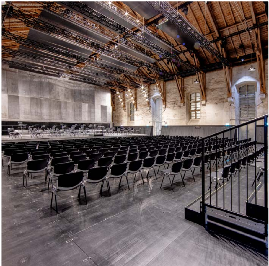
G-SORBER (einlagig / monocouche / single layer), Alte Reithalle – Aarau, Switzerland / Photos: © Hans-Jörg Huber Planungsbüro
