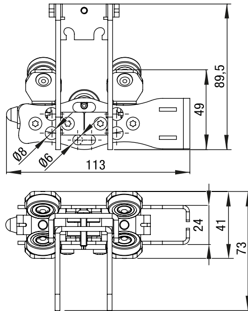
Abb. 14: Maße – Zugwagen für obenliegende Seilführung (OSF)
