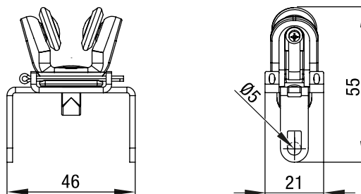
Abb. 9: Maße – OFFICE-Laufwagen
