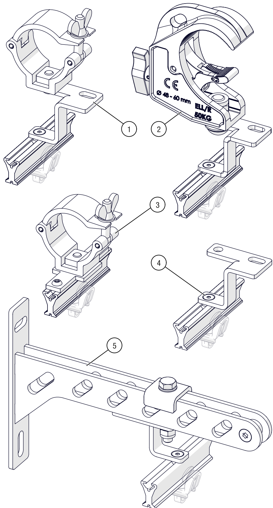
Abb. 6: G-TRACK – Abhängungsvarianten (2/2)
