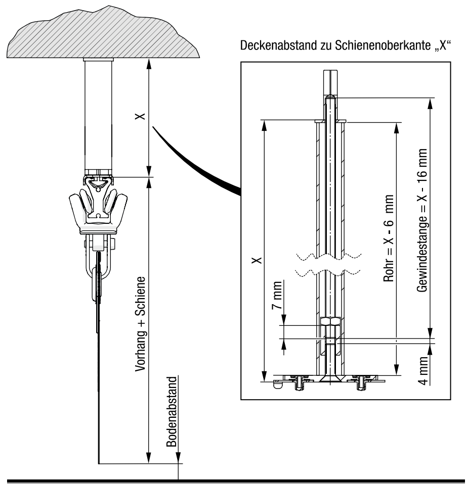
Abb. 22: Formeln zur Ermittlung von notwendiger Rohr- und Gewindestangenlänge
