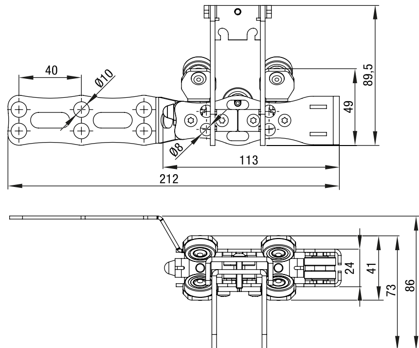
Abb. 15: Maße – Zugwagen für obenliegende Seilführung (OSF) mit Überzugbügel
