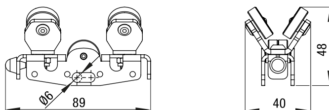
Abb. 10: Maße – Zugwagen
