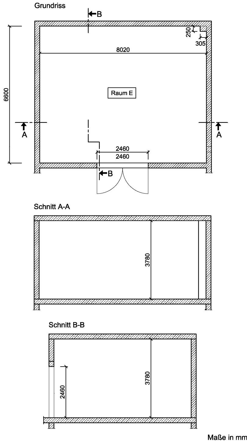
Abbildung C.1. Grundriss und Schnitte des Hallraums.
