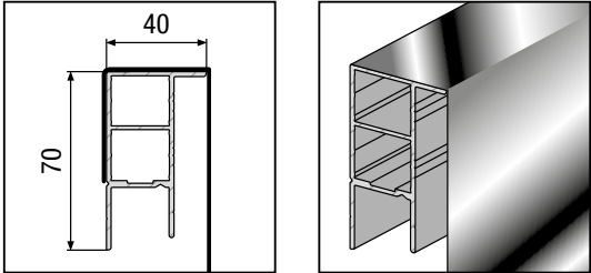
Rahmen / Cadre / Frame: 4 cm (1 ½")
