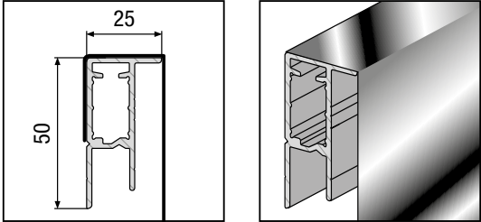
Rahmen / Cadre / Frame: 2,5 cm (1")
