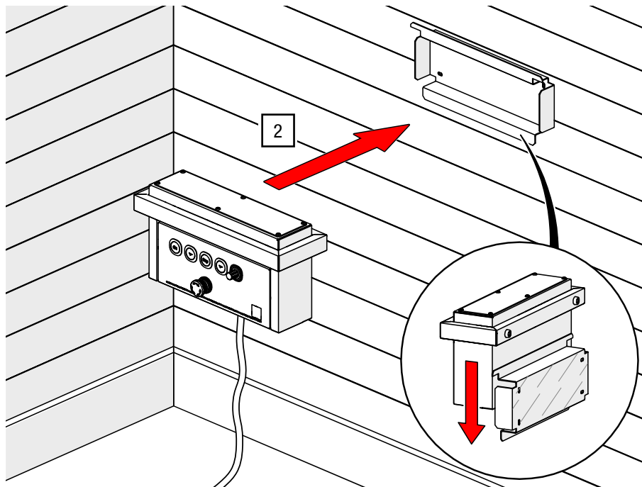
Abb. 27: 2. Bedienstelle aufhängen
