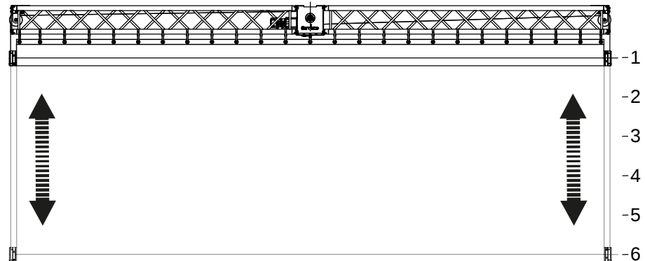
Abb. 4: Rollbildleinwand MEGASCREEN S – Endschalter und Notendschalter
